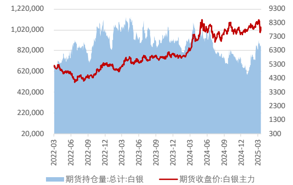
图表 20 白银期货持仓量
